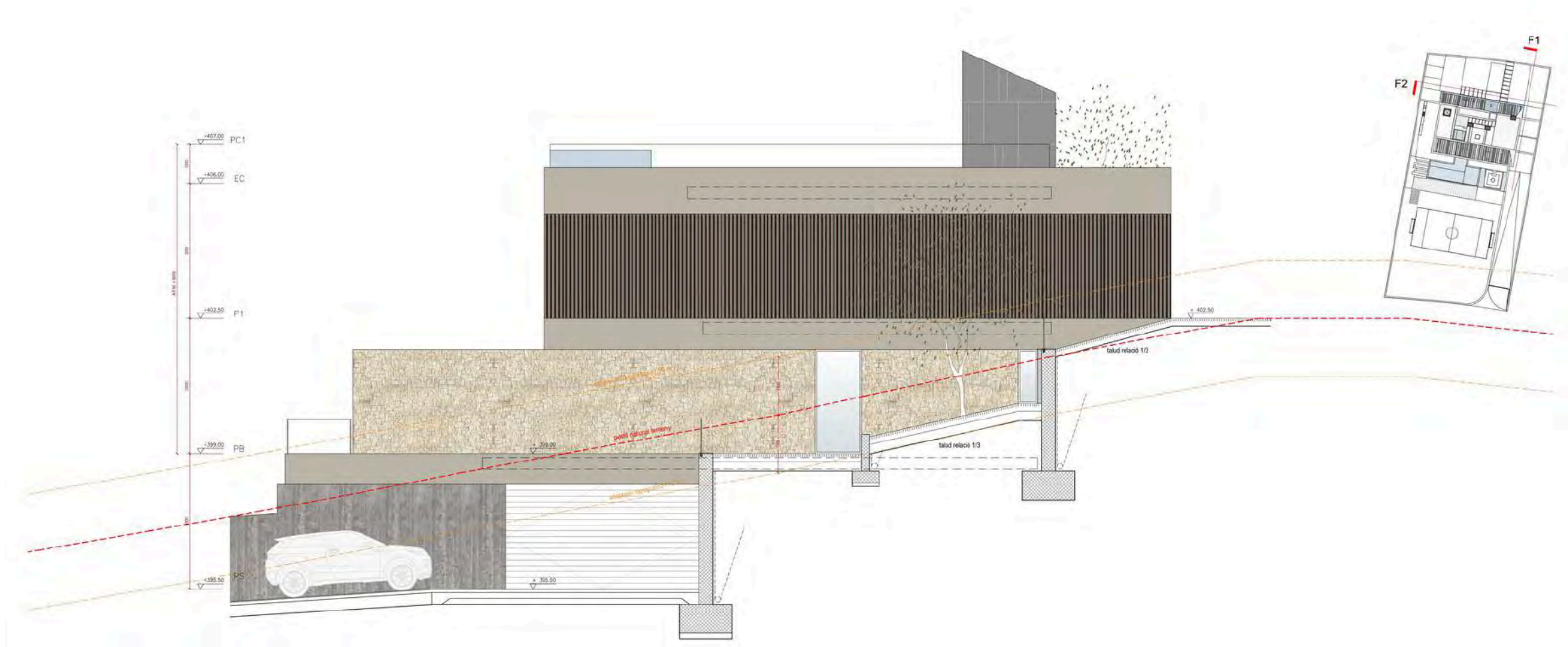
FAÇANA 1
